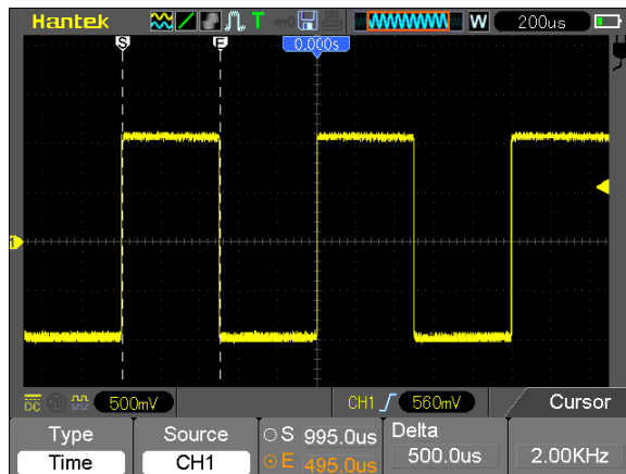
Курсор Time
