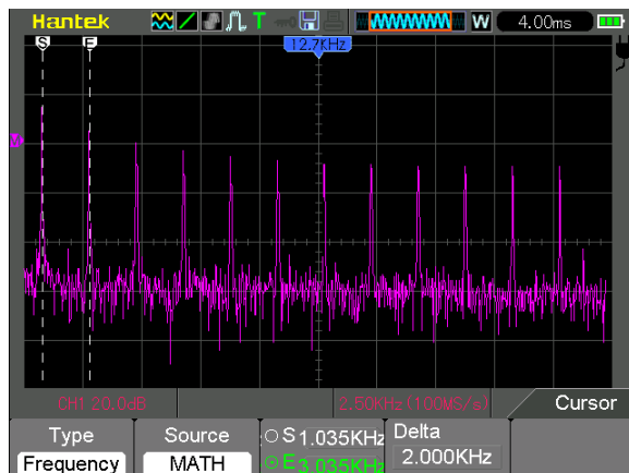
Курсоры частоты
