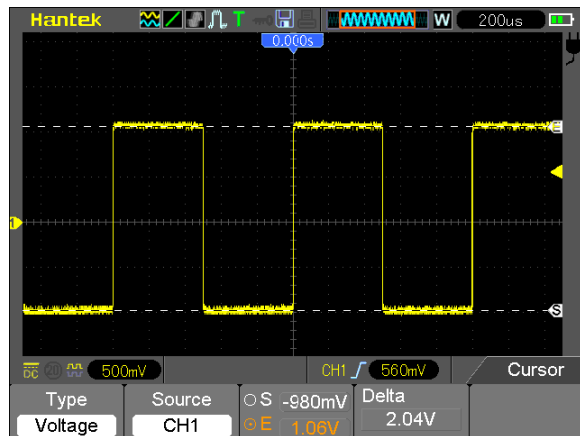
Курсор Voltage
