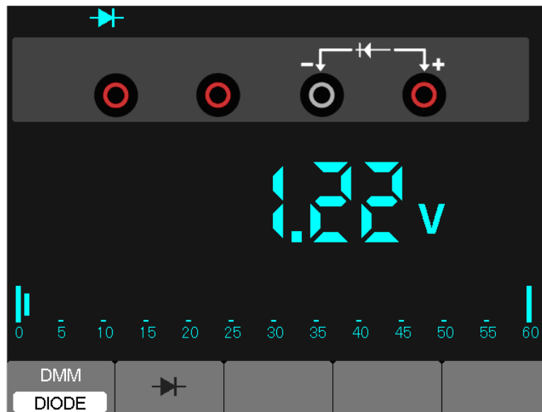
Рисунок 7-3 Диодное измерение
