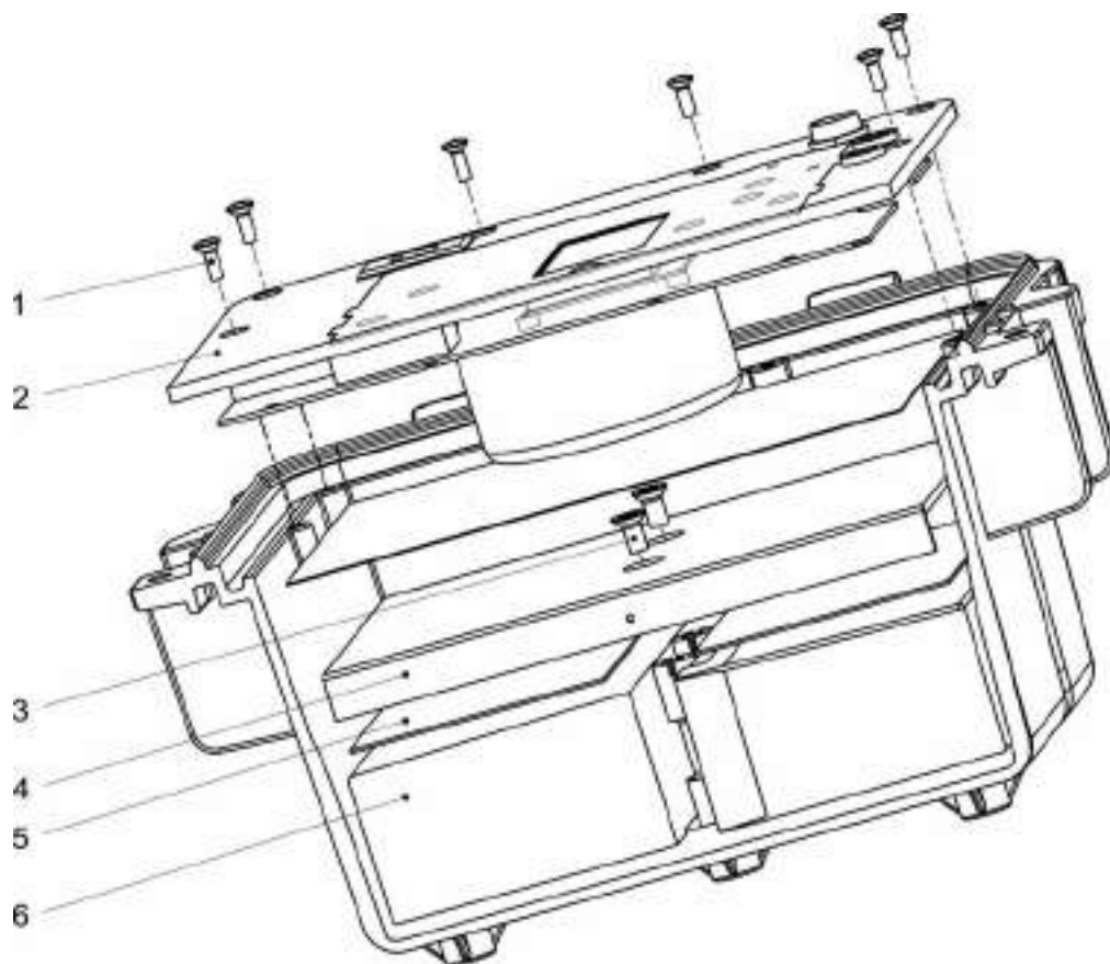
Рисунок 3.1 – Замена аккумуляторов
