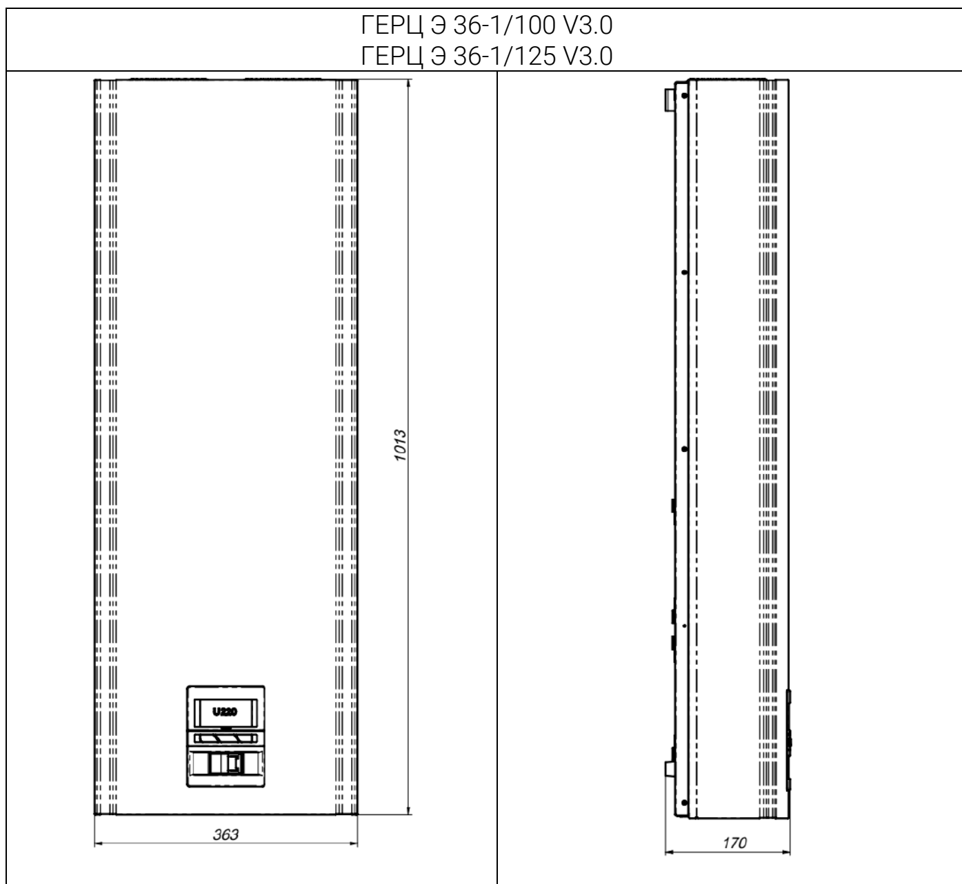
Рисунок 8. Габаритные размеры стабилизаторов Герц на 100-125А
