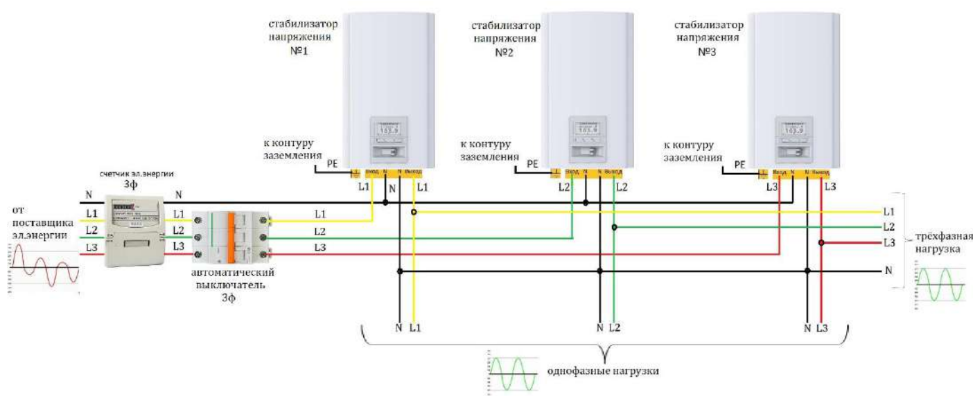
Рисунок 10. Схема подключения стабилизатора к трёхфазной сети
