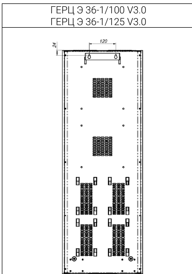
Рисунок 6. Установочные размеры стабилизаторов Герц на 100-125 А
