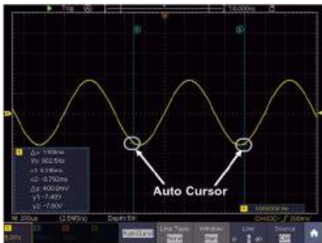
Рисунок 5-27 Автоматические курсоры
