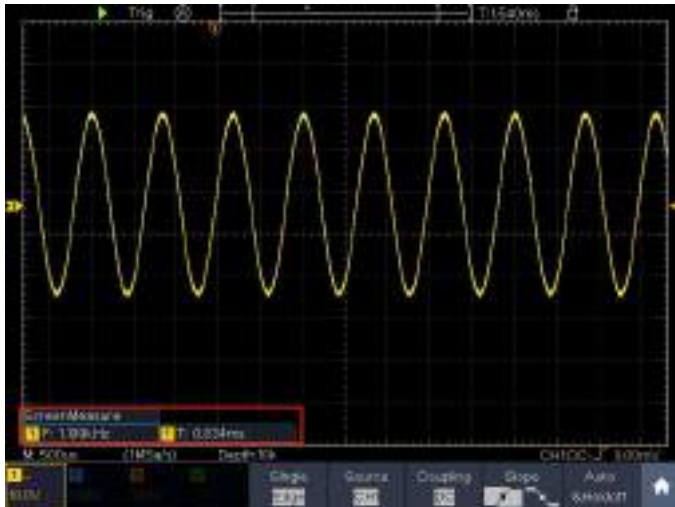
Рисунок 9-1 Измерения периода и частоты для данного сигнала
