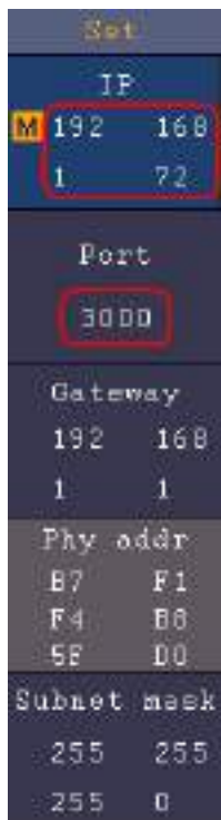
Рисунок 8-4 Установка параметров сети на осциллографе
