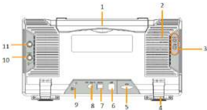
Рисунок 2-2 Задняя панель
