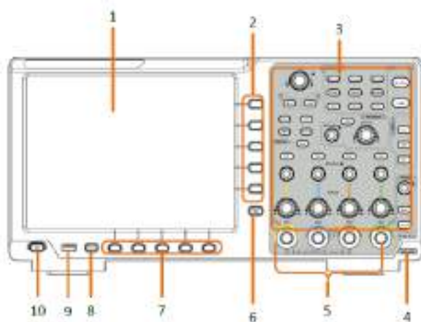
Рисунок 2-1 Передняя панель
