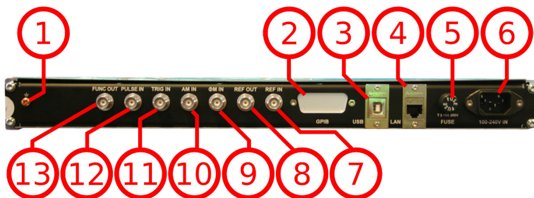
Рис.7:ВидзаднейпанелиAPSIN 1URM
