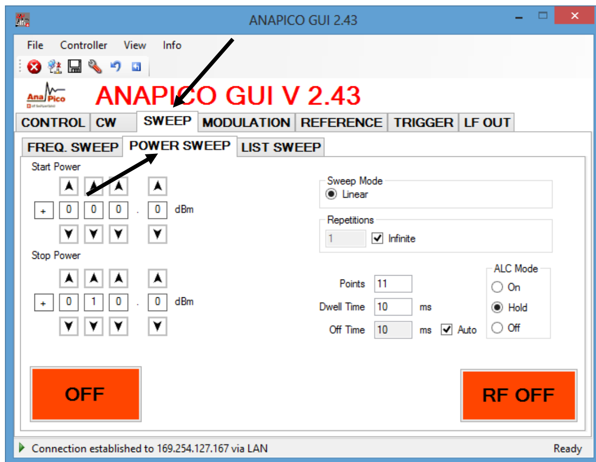
Рисунок 6-f. Вкладка «POWER SWEEP»
