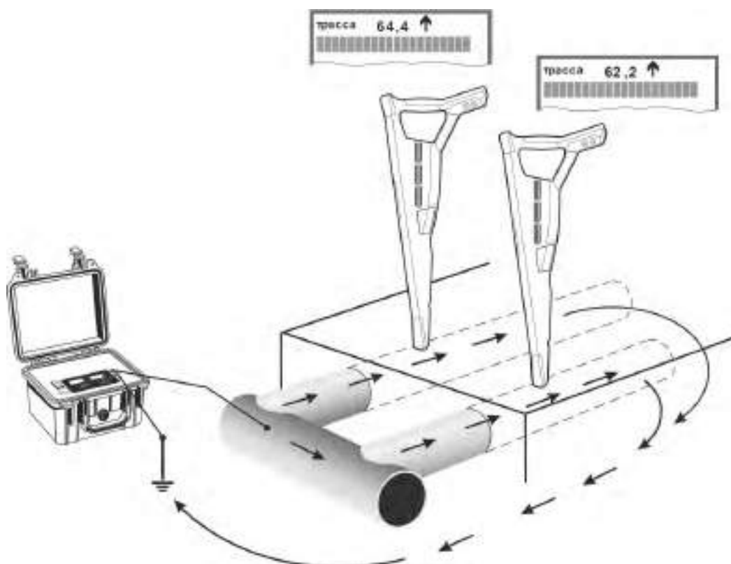
Рисунок 4.2.3.2 – Направление тока в гальванически связанных коммуникациях
