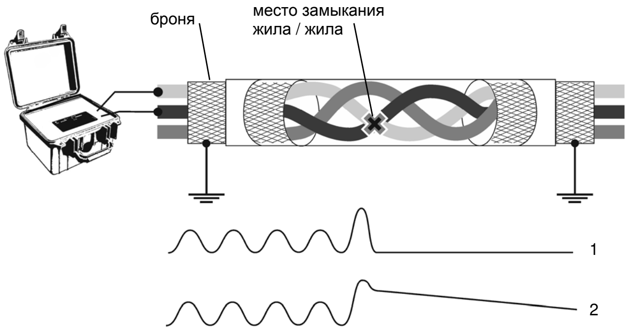
Рисунок 5.3.1 – Схема подключения и уровень сигнала при поиске замыкания между жилами
