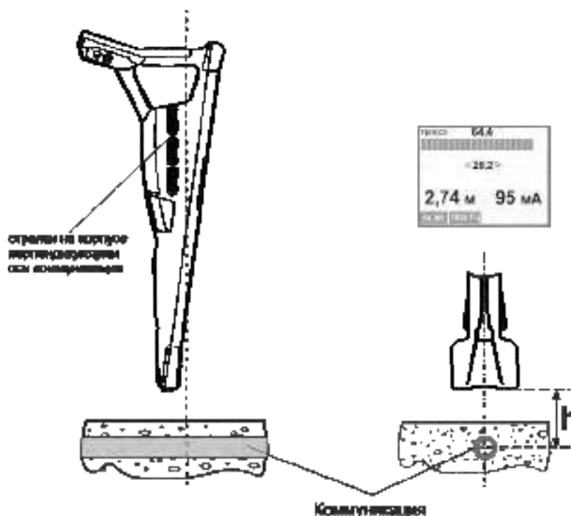
Рисунок 4.3 – Прямое определение глубины залегания
