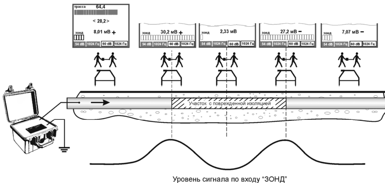
Рисунок 5.2.1 – Схема подключения и уровень сигнала при поиске повреждения изоляции по «минимуму»
