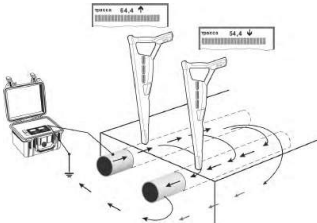
Рисунок 4.2.3.1 – Направление тока в соседней, гальванически развязанной коммуникации
