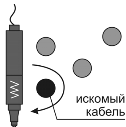
Рисунок 5.4.1 – Поиск кабеля (жилы) по максимуму сигнала
