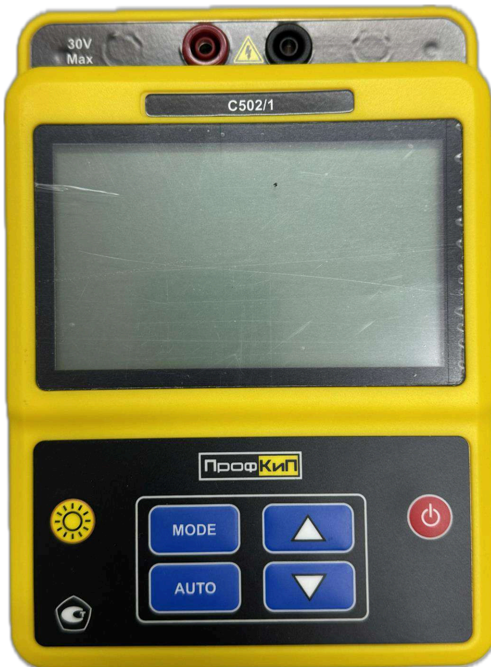
Рис.1 Внешний вид вольтметров ПрофКиП С502
